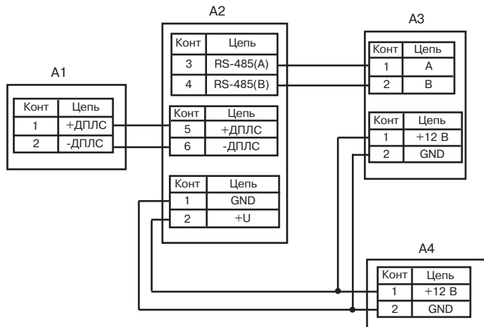
Рисунок 7 – Клеммы подключения
