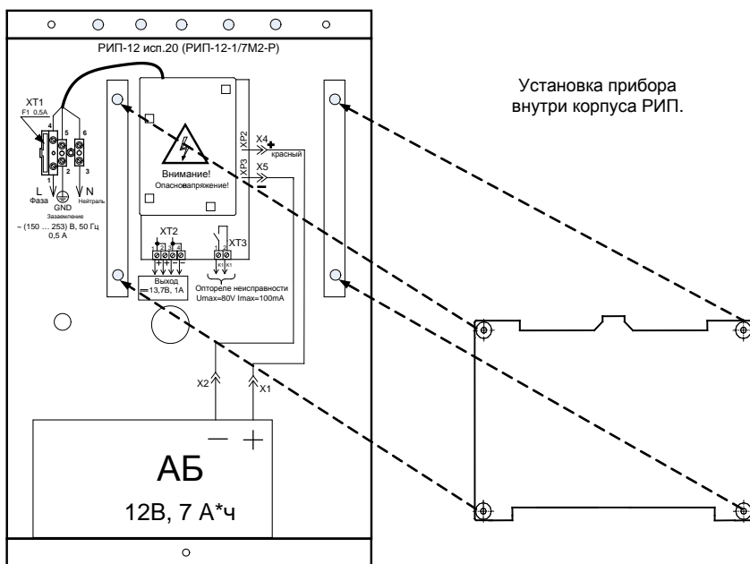
Рисунок 3. Установка прибора внутри корпуса РИП.
