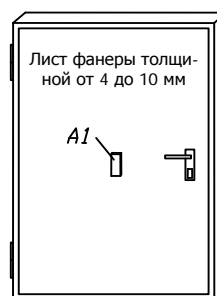
Рисунок 6. Защита деревянной пустотелой двери
