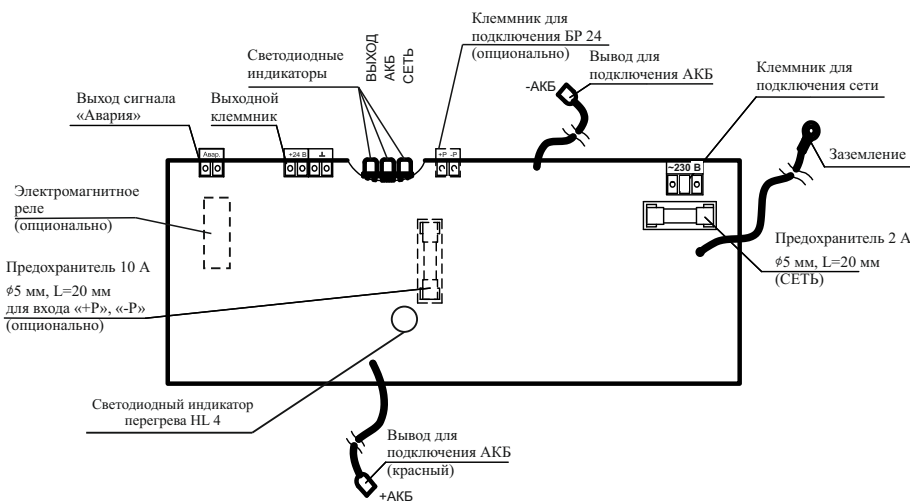
Рисунок 1 – Плата источника
