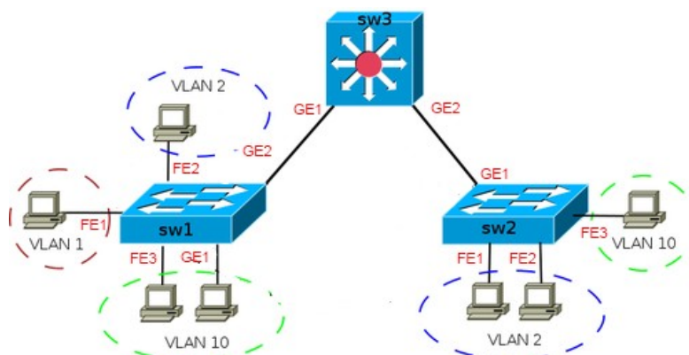
Рис. 5.3.14.1 Топология сети
